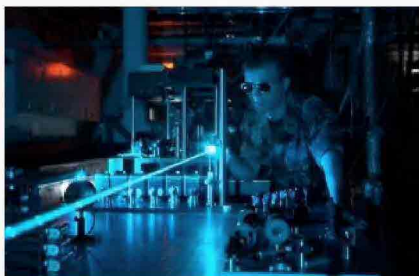
Fotoni emessi da un laser in un fascio coerente (fonte: Aeronautica degli Stati Uniti)
